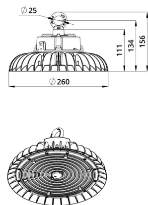
Габаритный чертеж
