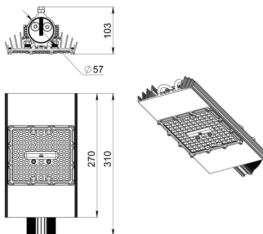
Габаритный чертеж
