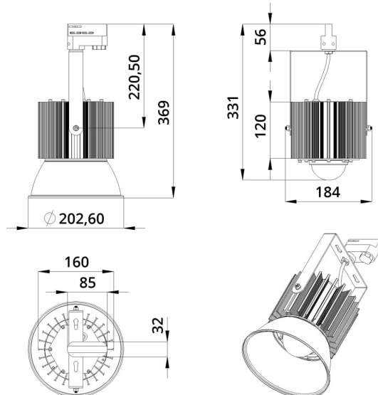
Габаритный чертеж
