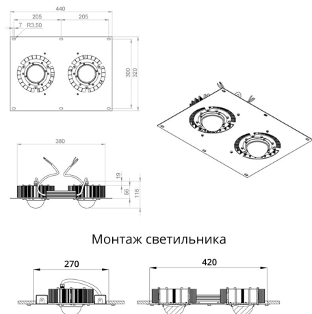
Габаритный чертёж
