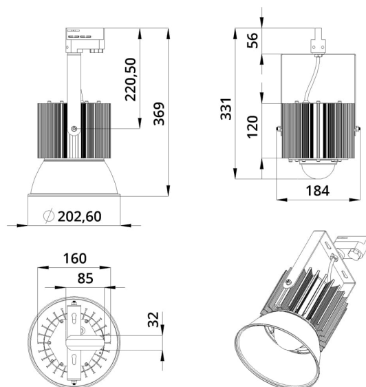
Габаритный чертеж
