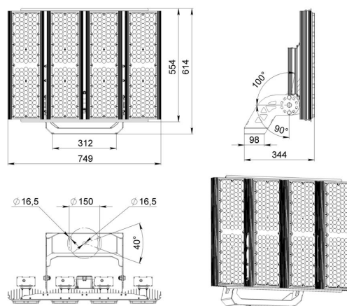
Габаритный чертеж
